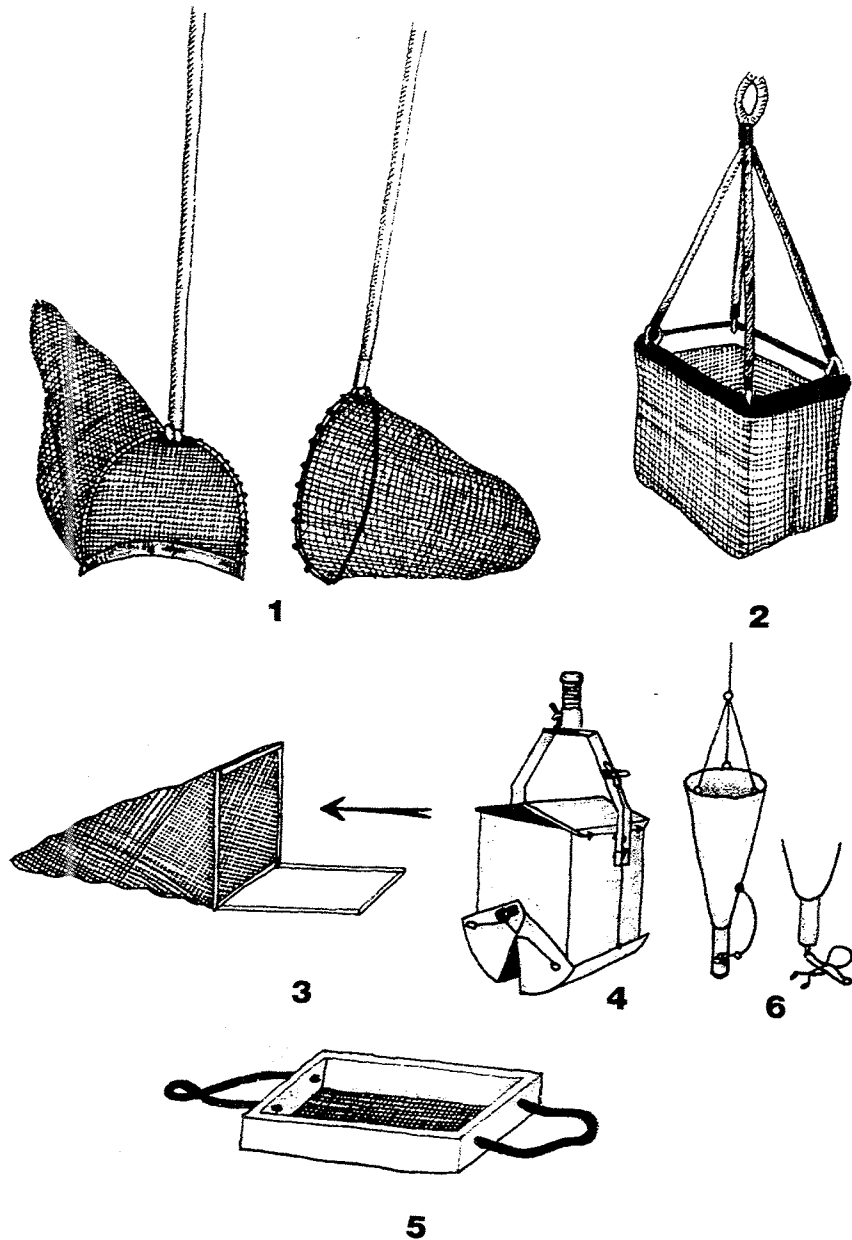
Sl. 26. OPREMA I PRIBOR KOJI KORISTIMO PRILIKOM ISTRAŽIVANJA KOPNENIH VODA: 1. bentos mreže, 2. dredža, 3. Surberova mreža, 4. grabilo (bager), 5. sito za ispiranje uzoraka dna, 6. planktonska mreža, 7. kraj za izradu planktonske mreže, 8. dubinska boca, 9. Secchi - disk, 10. boce širokog grla, 11. Petrijeva zdjelica
