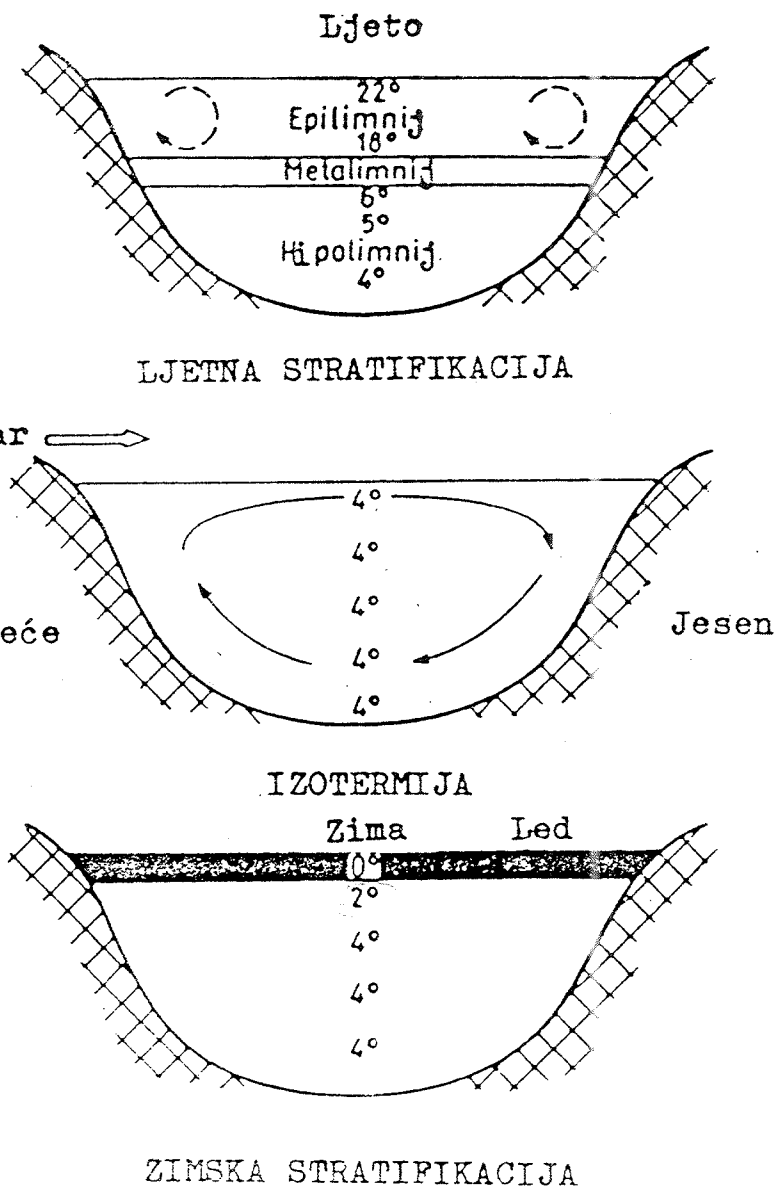
Sl. 2. TEMPERATURA I CIRKULACIJA VODE JEZERA UMJERENOG POJASA TIJEKOM GODINE
